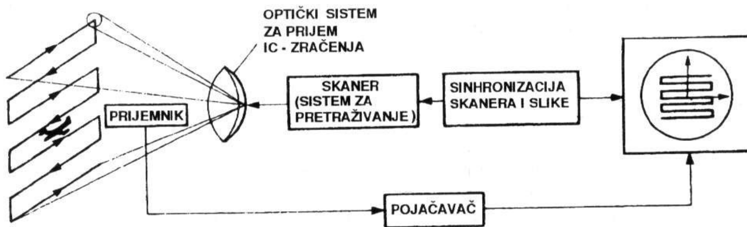
Slika 21.29. Princip termovizijskog sistema sa skeniranjem
